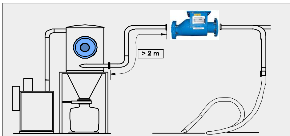
Всасывающий агрегат
